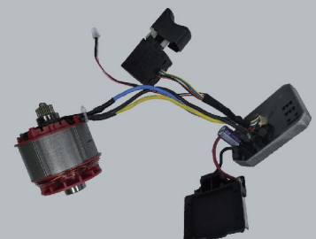
MOTOR SET
